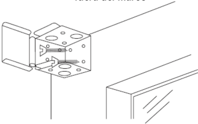
Montaje por fuera del marco
