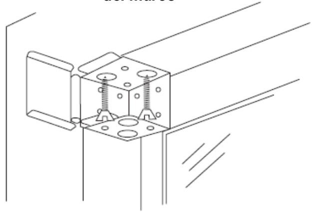
Montaje por dentro del marco
